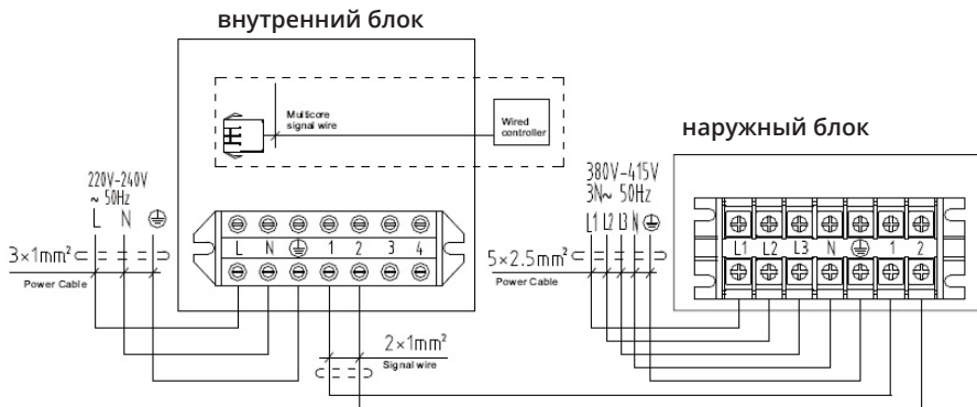
Схема для моделей LAC -36AC, LAC -48AC, LAC -60AC
