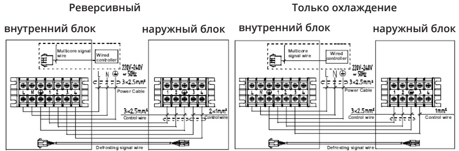
Схема для модели LAC -18AC
