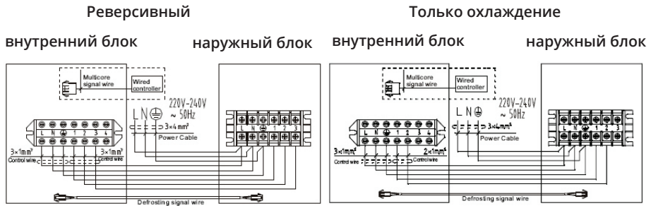
Схема для модели LAC -24AC
